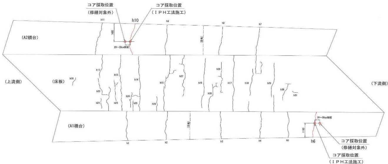
神社橋 補修図
